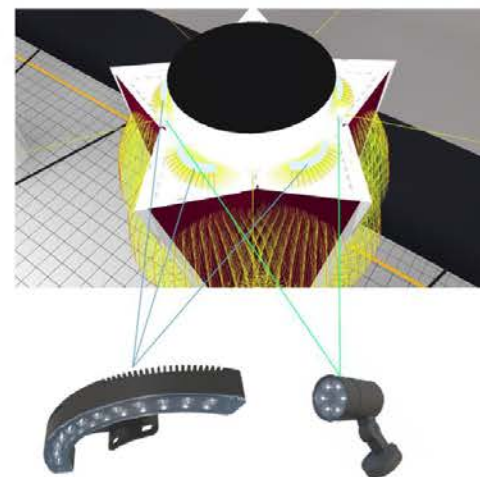
Даунлайт центр и край Схема размещения светильников на опоре
